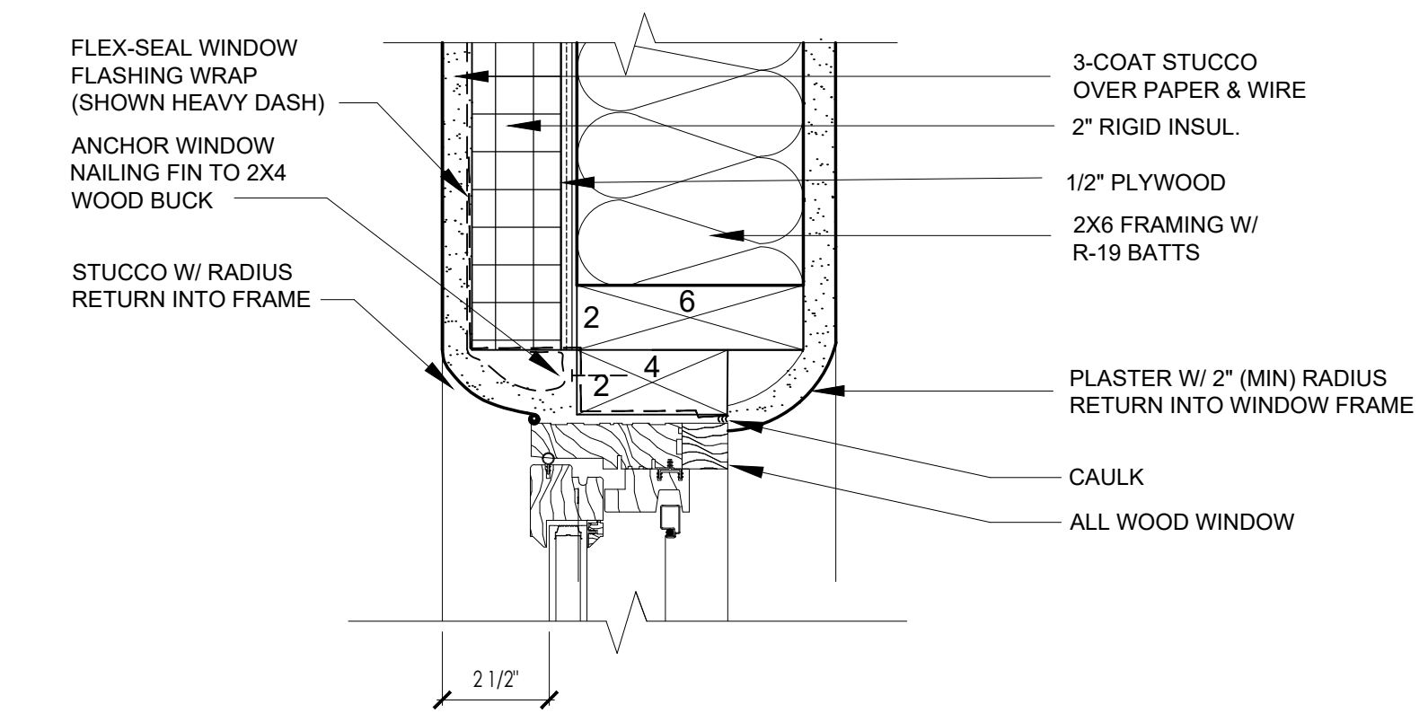
JAMB
